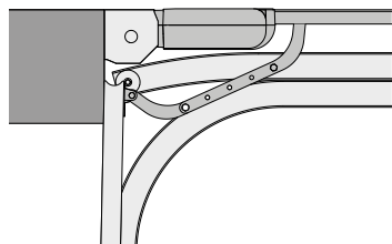
Installazione su albero portamolle
