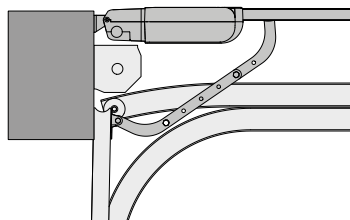
Installazione su architrave
